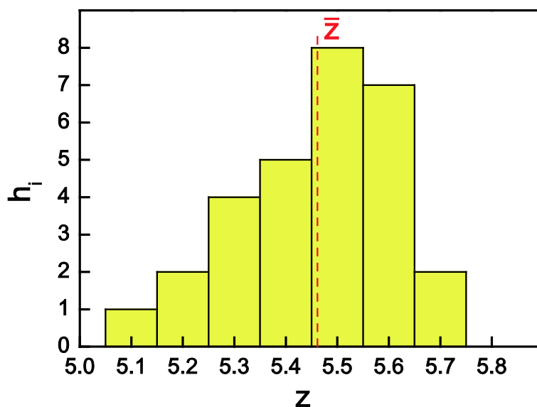
Abbildung 1: Histogramm
